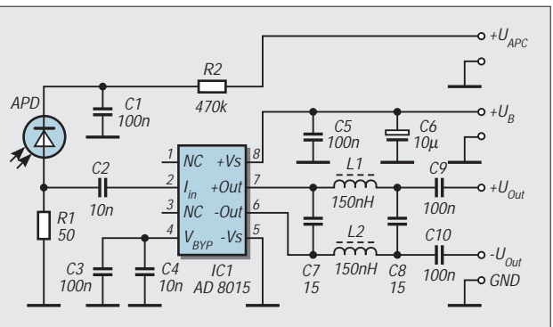
Bild 14: Zur Verstärkung des ADP-Signals wird der AD-Schaltkreis AD8015 verwendet.
