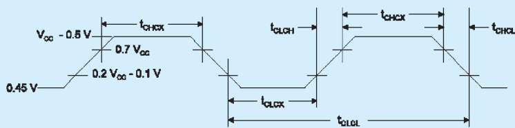
Bild 2: External Clock
