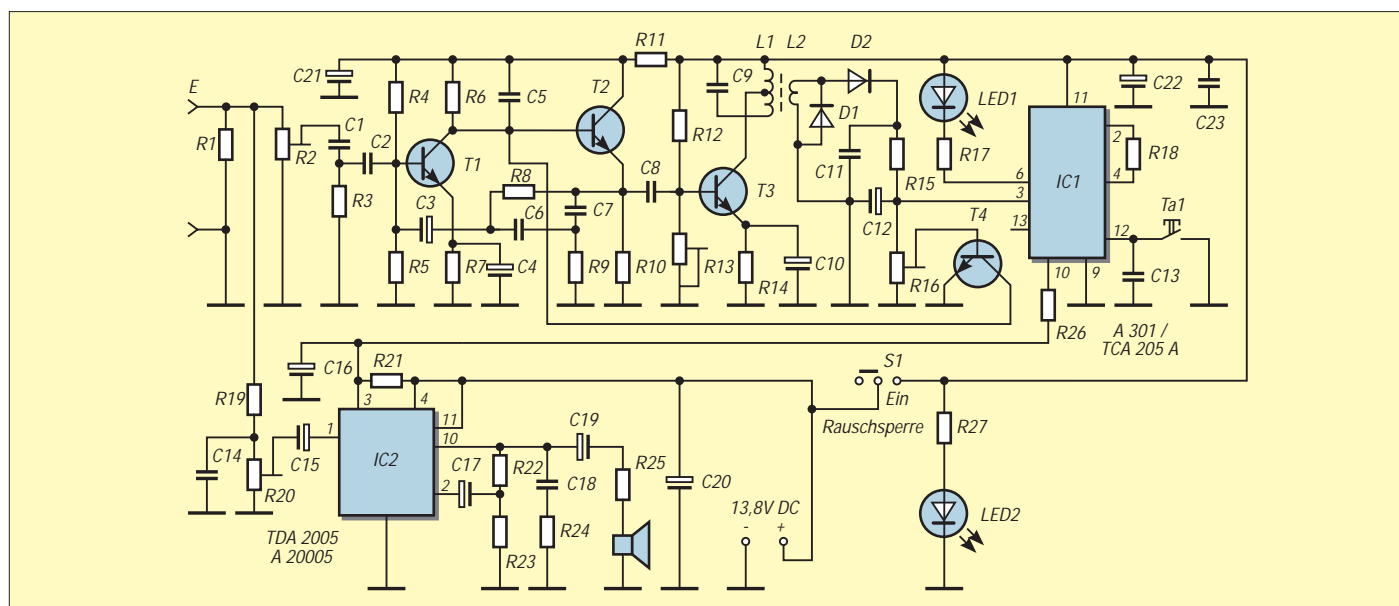
Bild 1: Stromlaufplan
