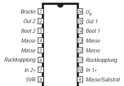
Bild 2: Anschlußbelegung des Powerdip-Gehäuses
