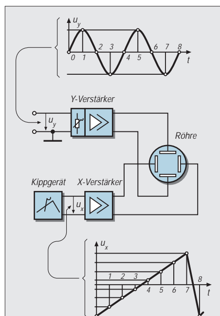
Bild 1: Schaltschema für ein Oszilloskop für die Darstellung periodisch ablaufender Zeitfunktionen. An den X-Platten liegt eine zeitlinear verlaufende Ablenkspannung, an den Y-Platten die darzustellende Meßspannung (hier eine sinusförmige) Wechselspannung.
