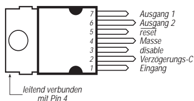
Bild 2: Pinbelegung des siebenpoligen Gehäuses mit Kühlfahne
