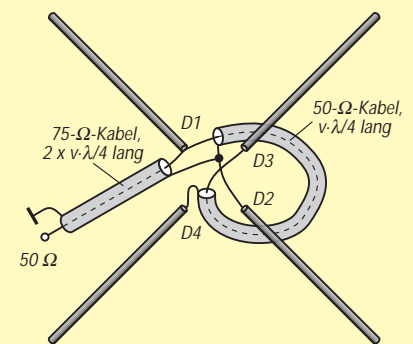
Bild 4: Schema der Zusammenschaltung von Phasen- und Anpaßleitung bei der 2-Element-Yagi
