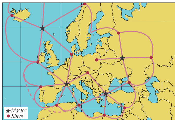
Loran-C-Stationen, Master und Slaves, im europäischen Bereich mit Reichweitenangaben
