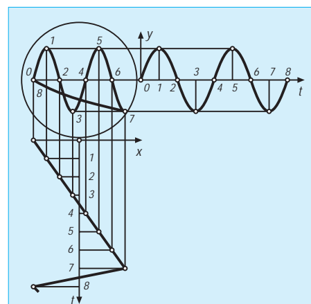
Bild 2: Zeichnerische Konstruktion der auf dem Bildschirm entstehenden Abbildung für die im Bild 1 an den Verstärkern des Oszilloskops anliegenden Spannungen. Die dünnen Konstruktionshilfslinien zeigen, für gleich weite Zeitspannen numeriert, die Lage des Leuchtflecks zu diesen Zeiten auf dem Bildschirm.
