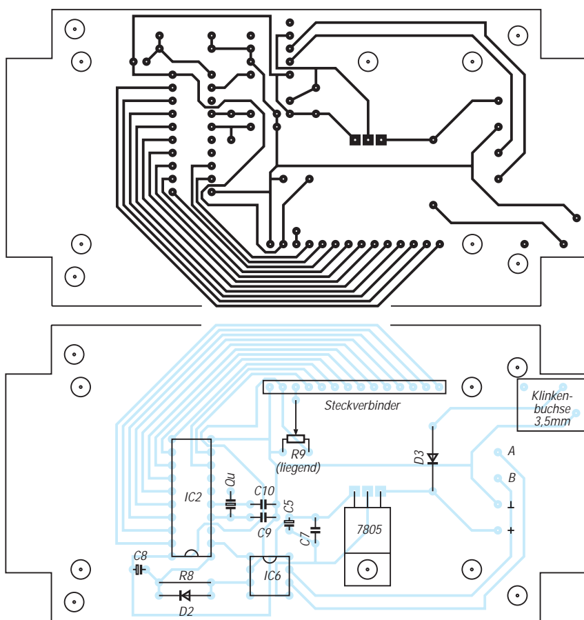
Bild 5: Platinenlayout des Empfangsteils
