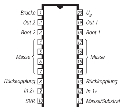
Bild 3: Anschlußbelegung des SMD-Gehäuses SO 20
